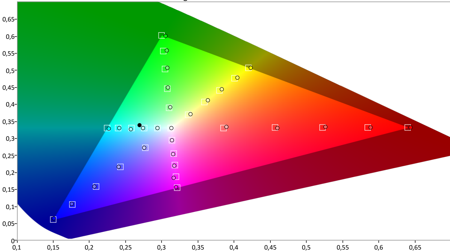
Diagramme de chromacité CIE
