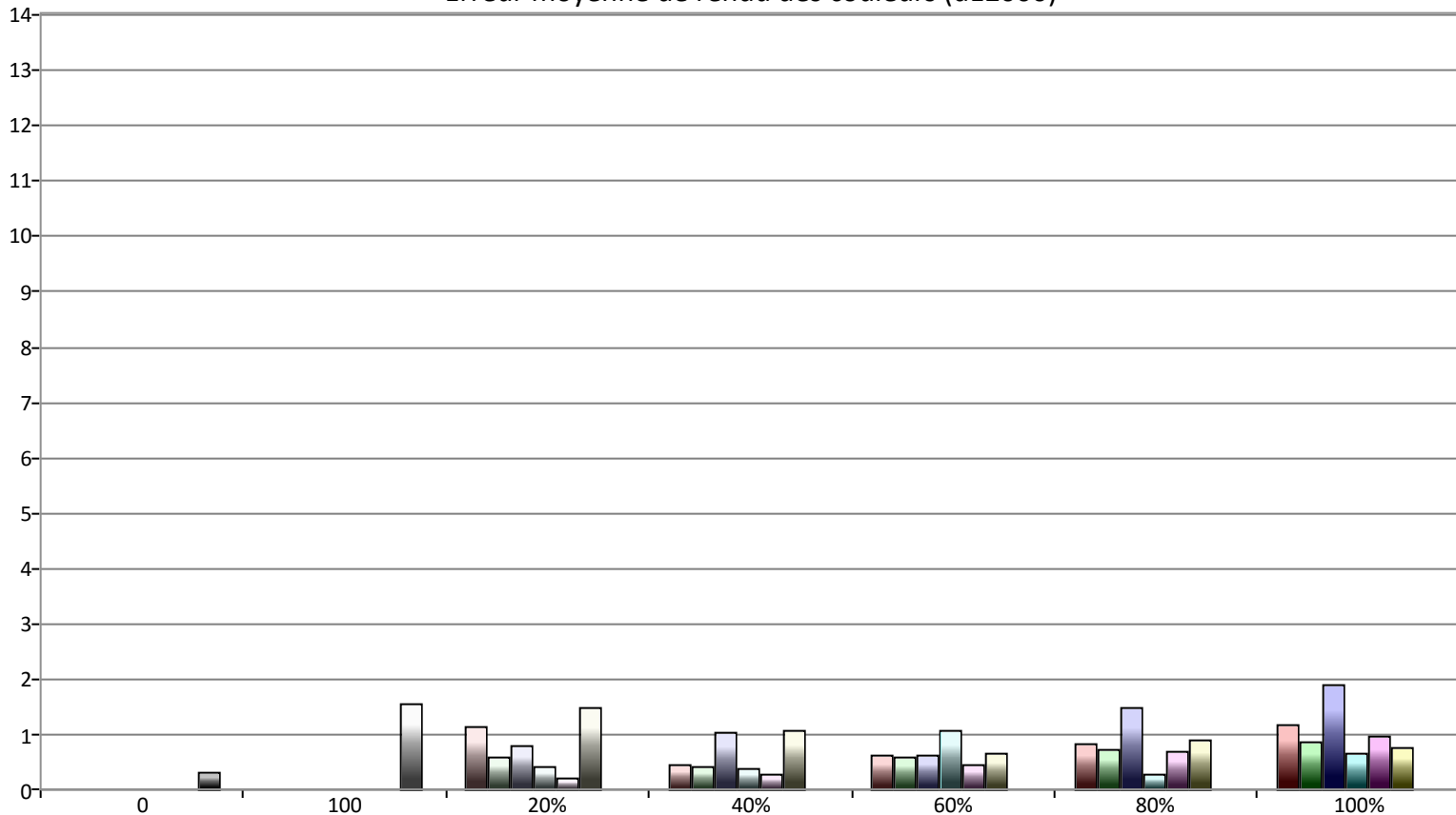
Erreur moyenne de rendu des couleurs (dE2000)
